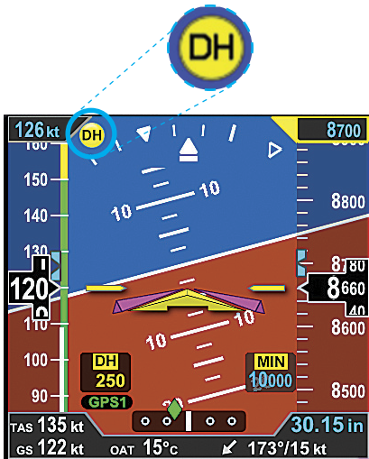
Figure 4-32 DH Annunciation
